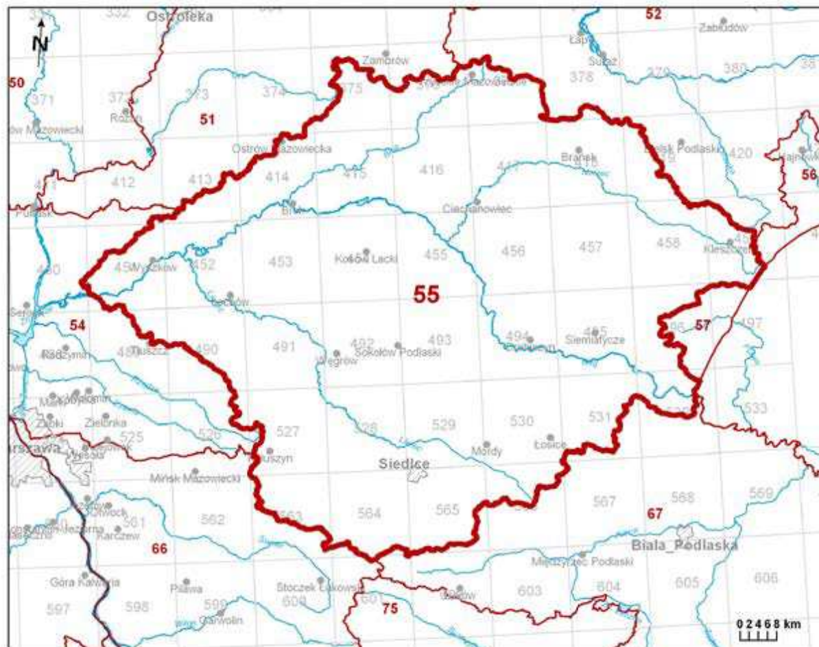
Rys. 7. Zasięg JCWPd 55.
