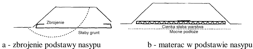
Rys. 2.2. Przykłady zbrojenia nasypów geosyntetykami
